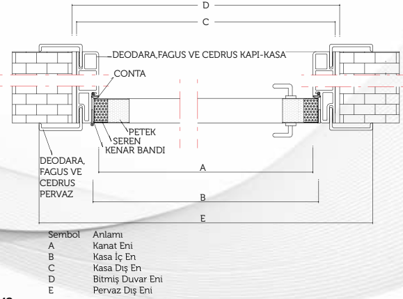
Kapı - Kasa Bağlantı Sistem Detayı
